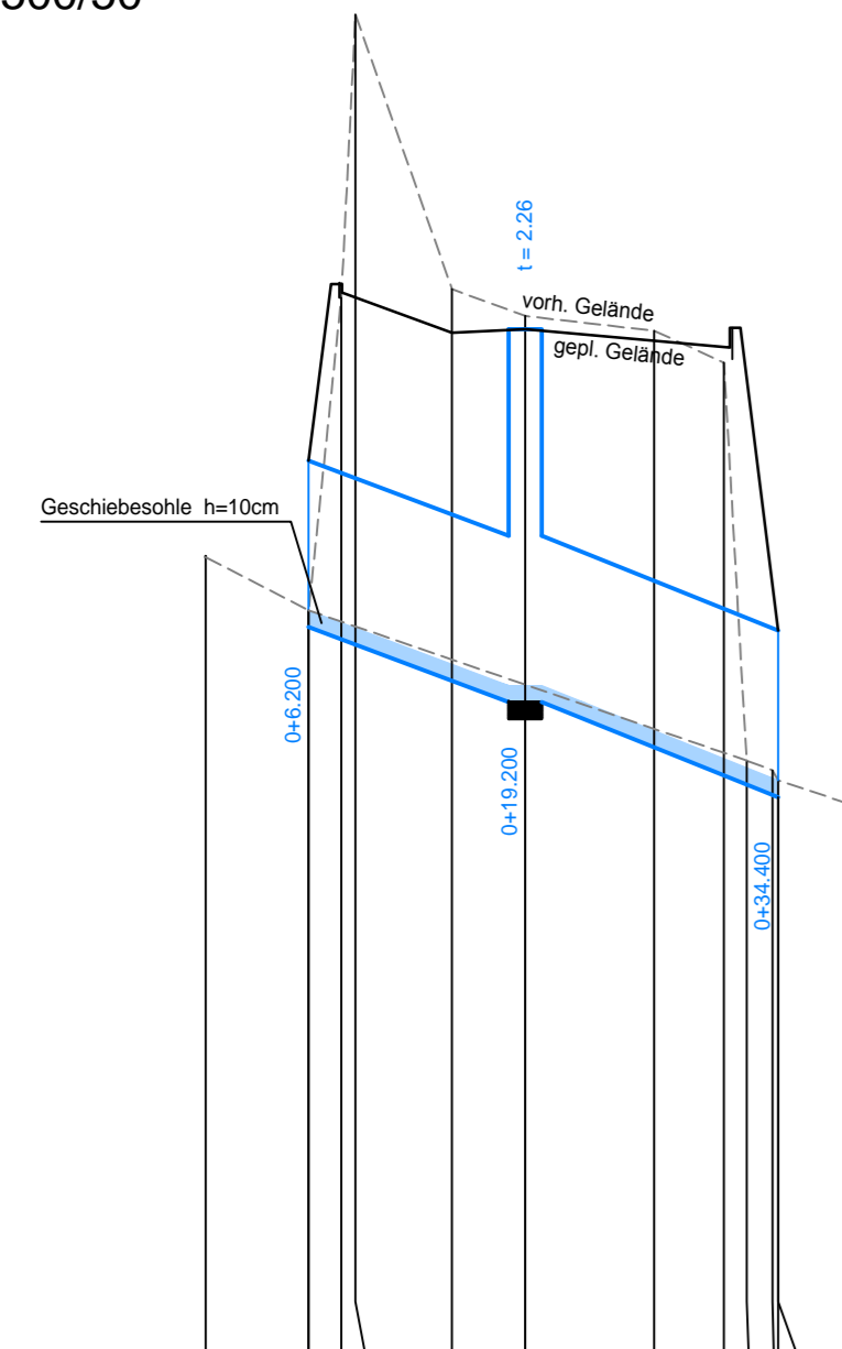
Längsschnitt Parzelle 49 M. 1:500/50
